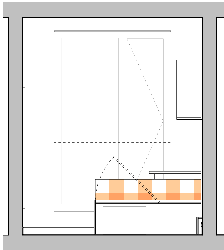
2 BEDROOM ELEVATION Scale: 1:25
